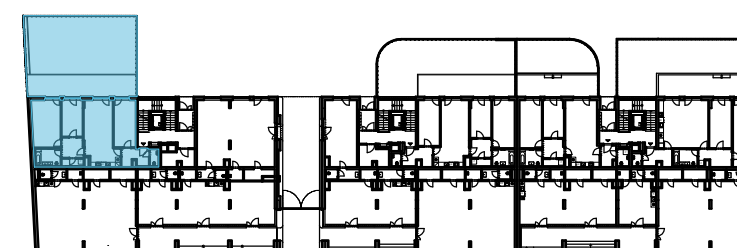
PŮDORYS 1.NP
